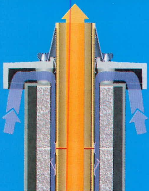
Ellenáramú működés. A fentről érkező levegő előmelegszi a belső cső felületén, növelve ezzel a fűtőberendezés hatásfokát.
