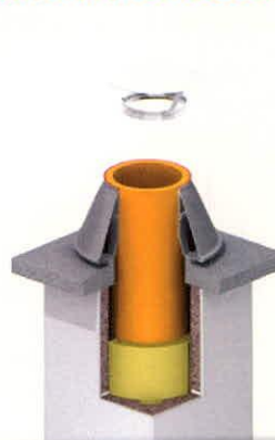
VAKOLT KÉMÉNYFEJ GYÁRI FEDLAPPAL
